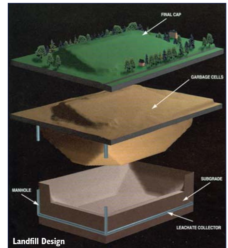
Landfill Design
